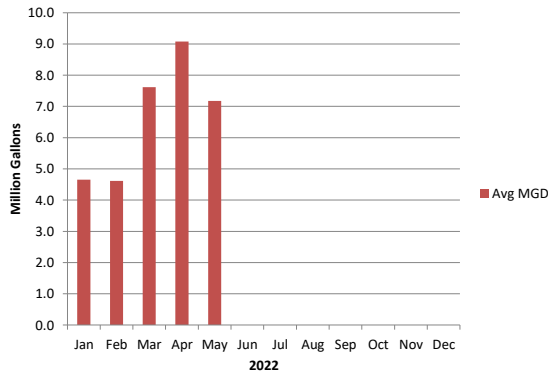
Avg Influent MGD/Mo.
